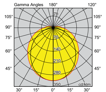
5FT/1500MM 56W 5000K
